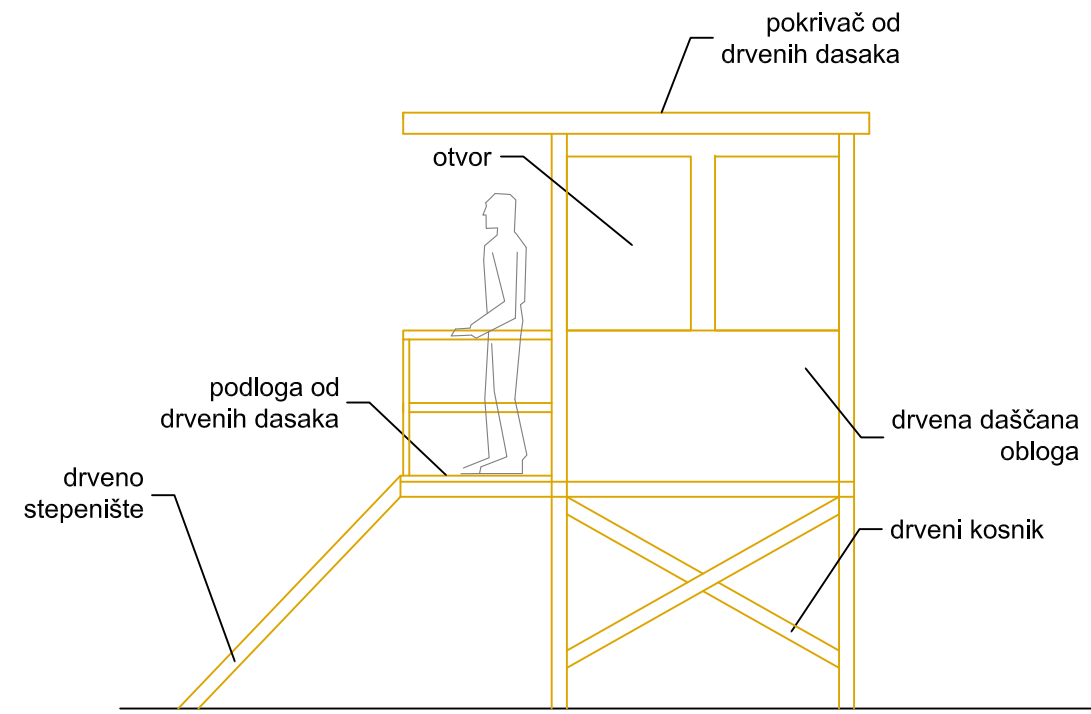
IZGLED A
